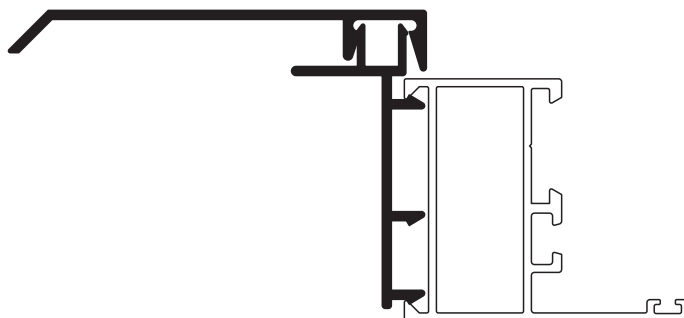
» MONTAJE JAMBA LISA «
