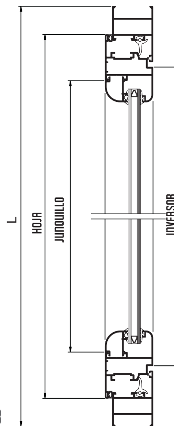
SECCIÓN B-B
