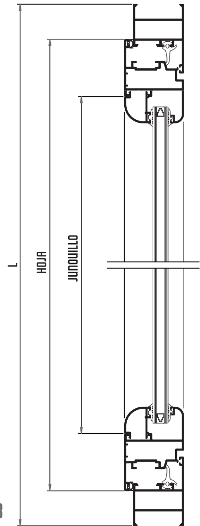
SECCIÓN B-B
