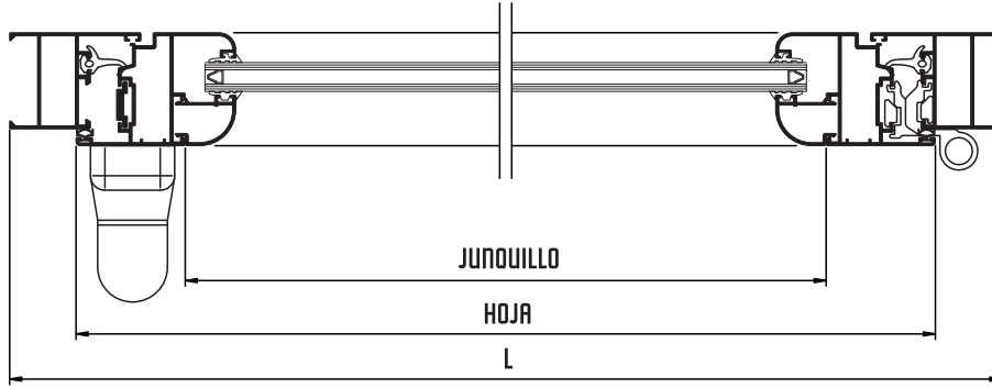
SECCIÓN A-A
