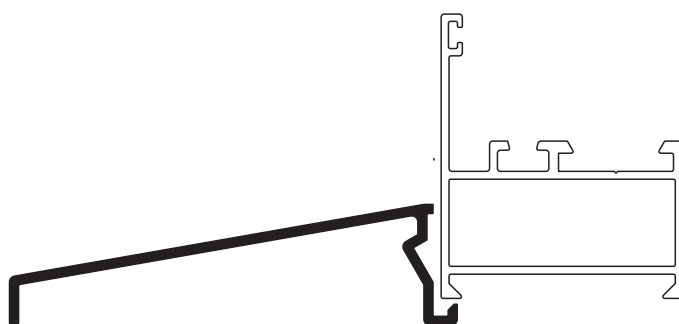
▶▶ MONTAJE GOTERÓN ▶▶
