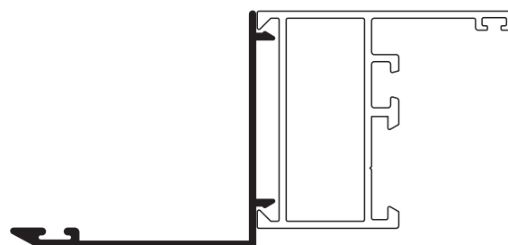
MONTAJE SOLAPE DE MARCO
