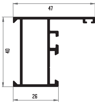
200 MARCO SIMPLE
