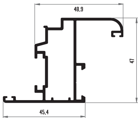
204 HOJA CURVA VENTANA
