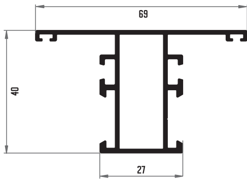
209 TRAVESAÑO VENTANA 69 MM
