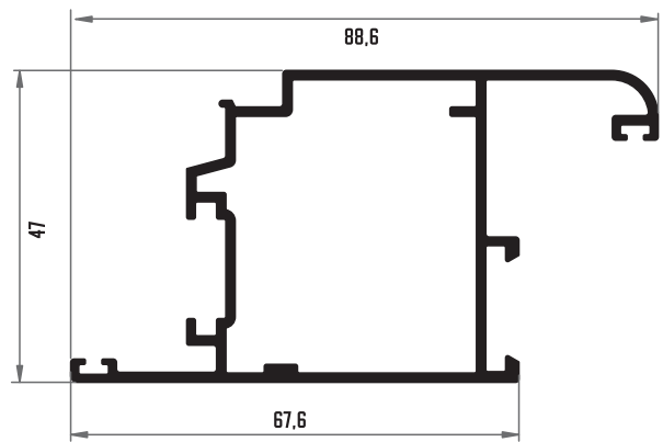
205 HOJA CURVA PORTADA
