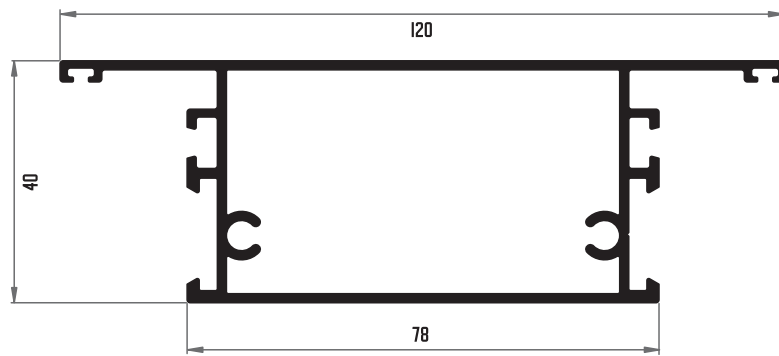
211 TRAVESAÑO DE ZÓCALO
