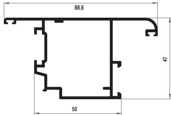
207 HOJA PORTADA APERTURA EXTERIOR
