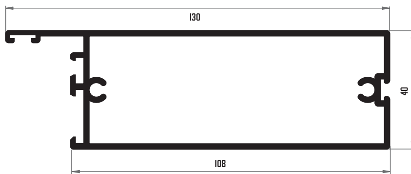
214 MARCO DE ZÓCALO
