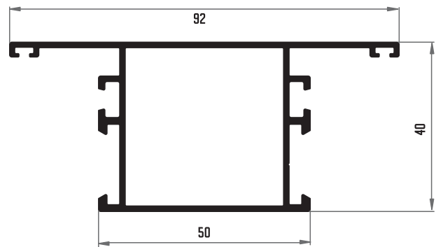
210 TRAVESAÑO PORTADA
