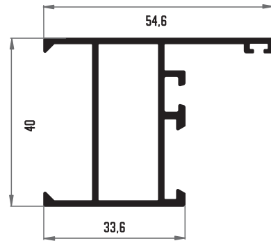
201 MARCO CON OREJAS
