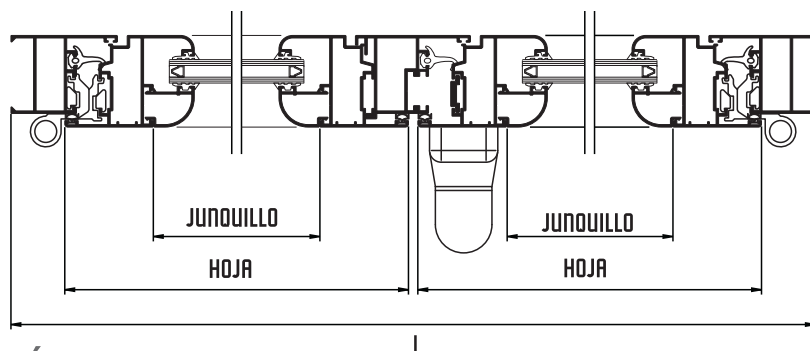
SECCIÓN A-A
