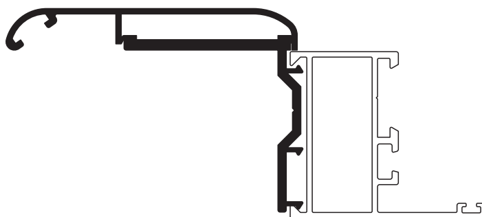
» MONTAJE JAMBA CURVA «
