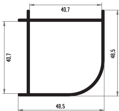
217 ESQUINERO 40 MM
