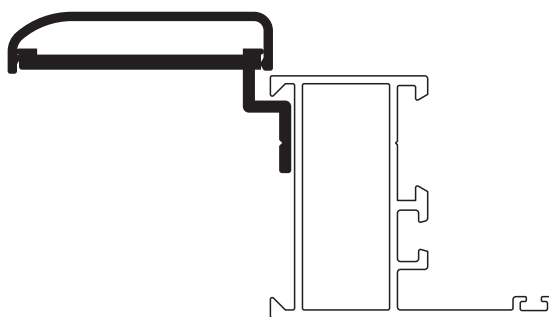
» MONTAJE JAMBA CURVA «
