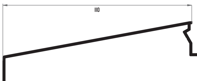
▶▶ 2770 GOTERÓN 110 mm ▶▶
