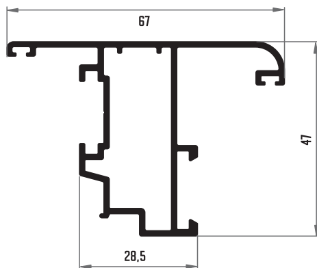
206 HOJA VENTANA APERTURA EXTERIOR
