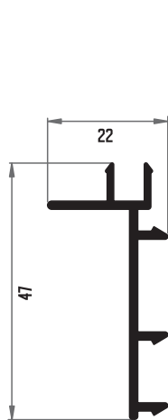
▶▶ 019 ACOUPLE PARA JAMBA LISA ▶▶
