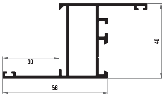
202 MARCO CON SOLAPE
