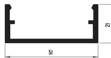
10003 ANCLAJE 51 MM
