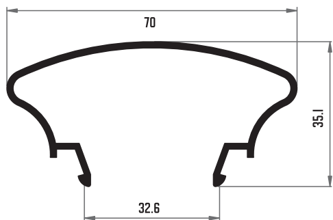
10022 PASAMANOS 70 MM
