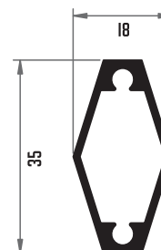
10006 TUBO 35X18 C/GUSANILLO
