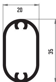
10005 TUBO OVALADO 35X20 C/GUSANILLO
