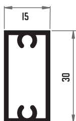
10020 BARRA BARANDILLA 30X15 MM
